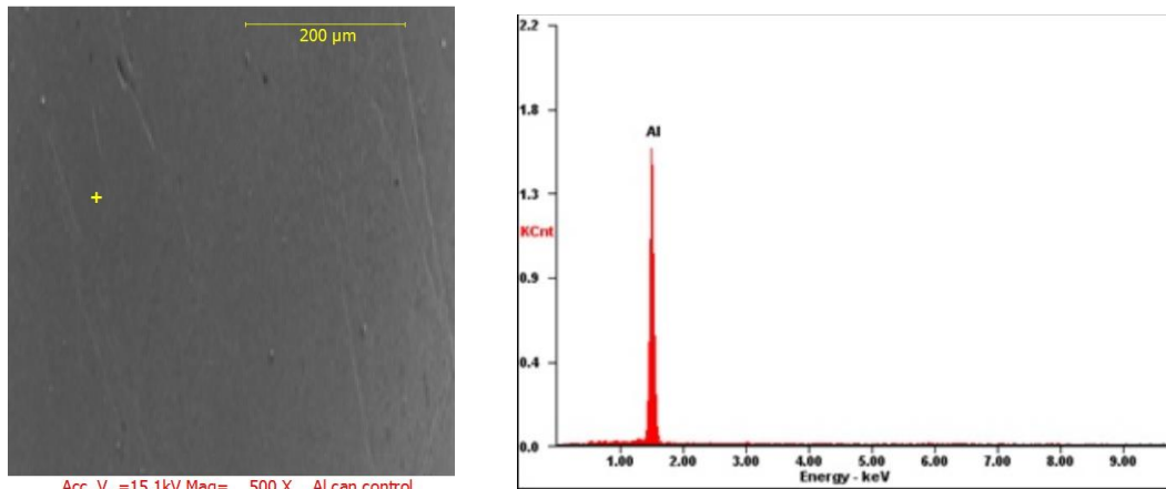
Fig 2: SEM/EDX of Al alloy (control)
